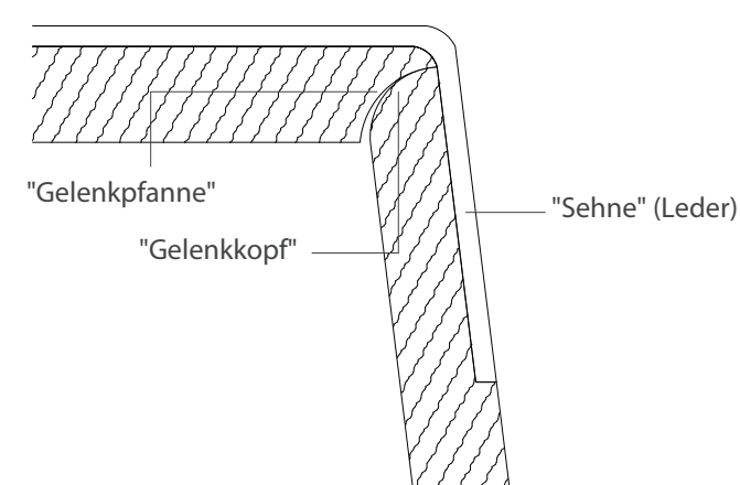
Gelenkverbindung 1:1
